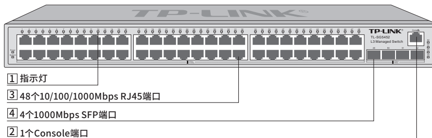
图1-1 TL-SG5452前面板示意图
